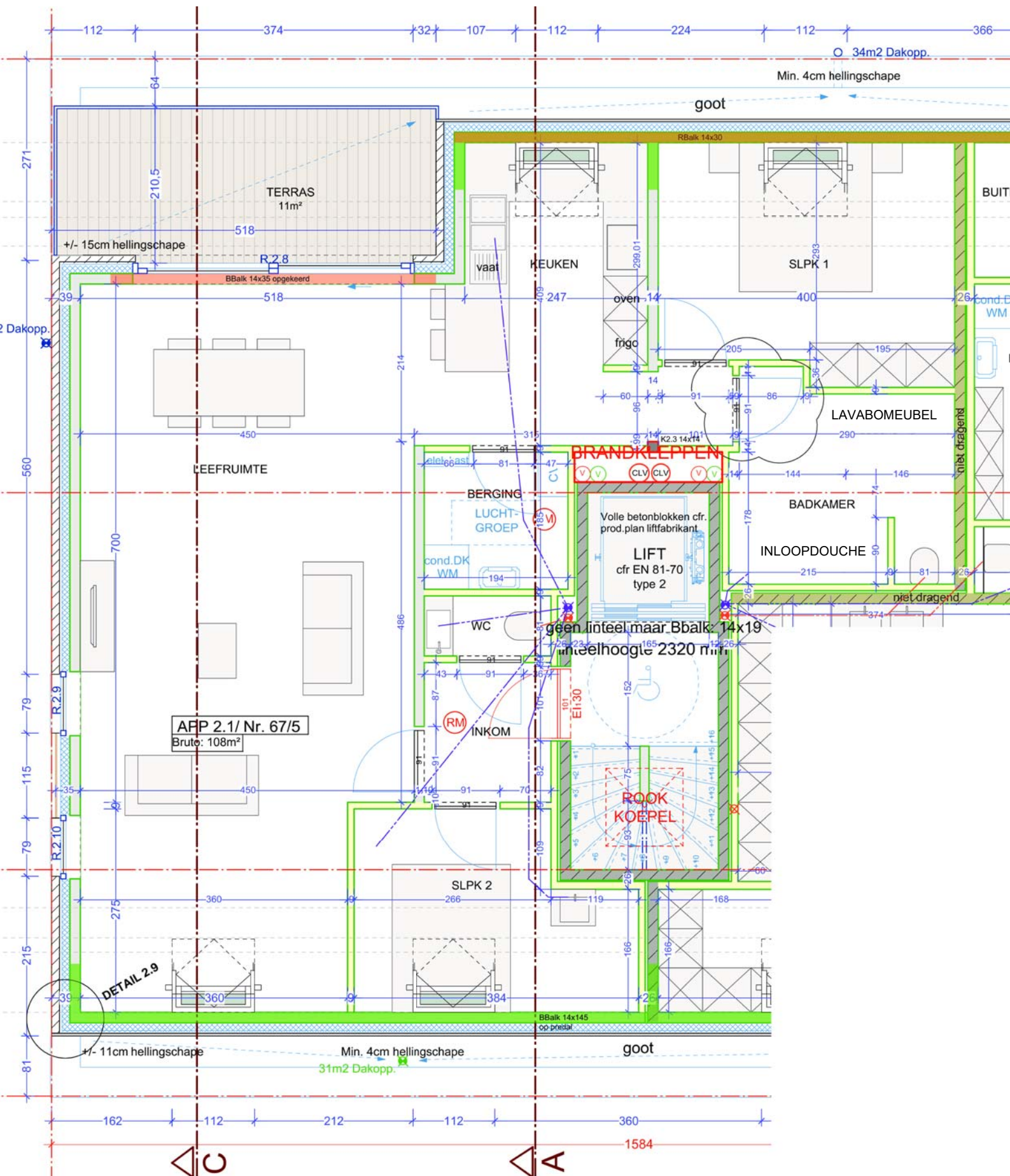
GRONDPLAN VERDIEPING +2 1/50
